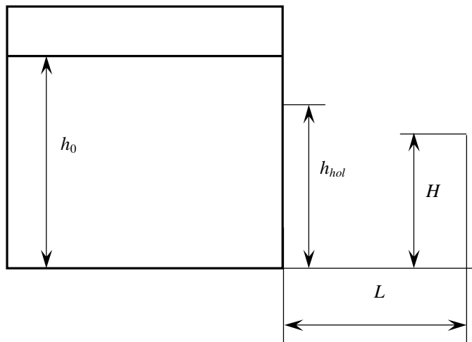
Рис. ПЗ.1. Схема для расчета истечения жидкости из отверстия в резервуаре
