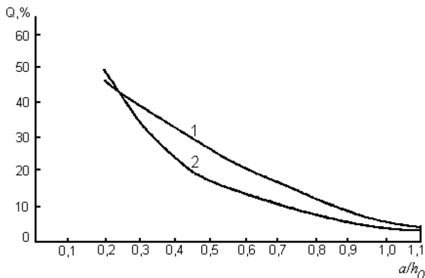
Рис. ПЗ.3. Зависимость доли перелившейся через обвалование жидкости Q от параметра a/h_0 : 1 - расчет; 2 - эксперимент
